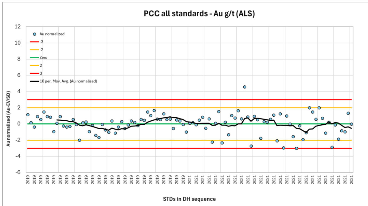
Figure 11-6: 2019-2021 PCC CRM Performance ALS – Au (Source: MMTS, 2025)
