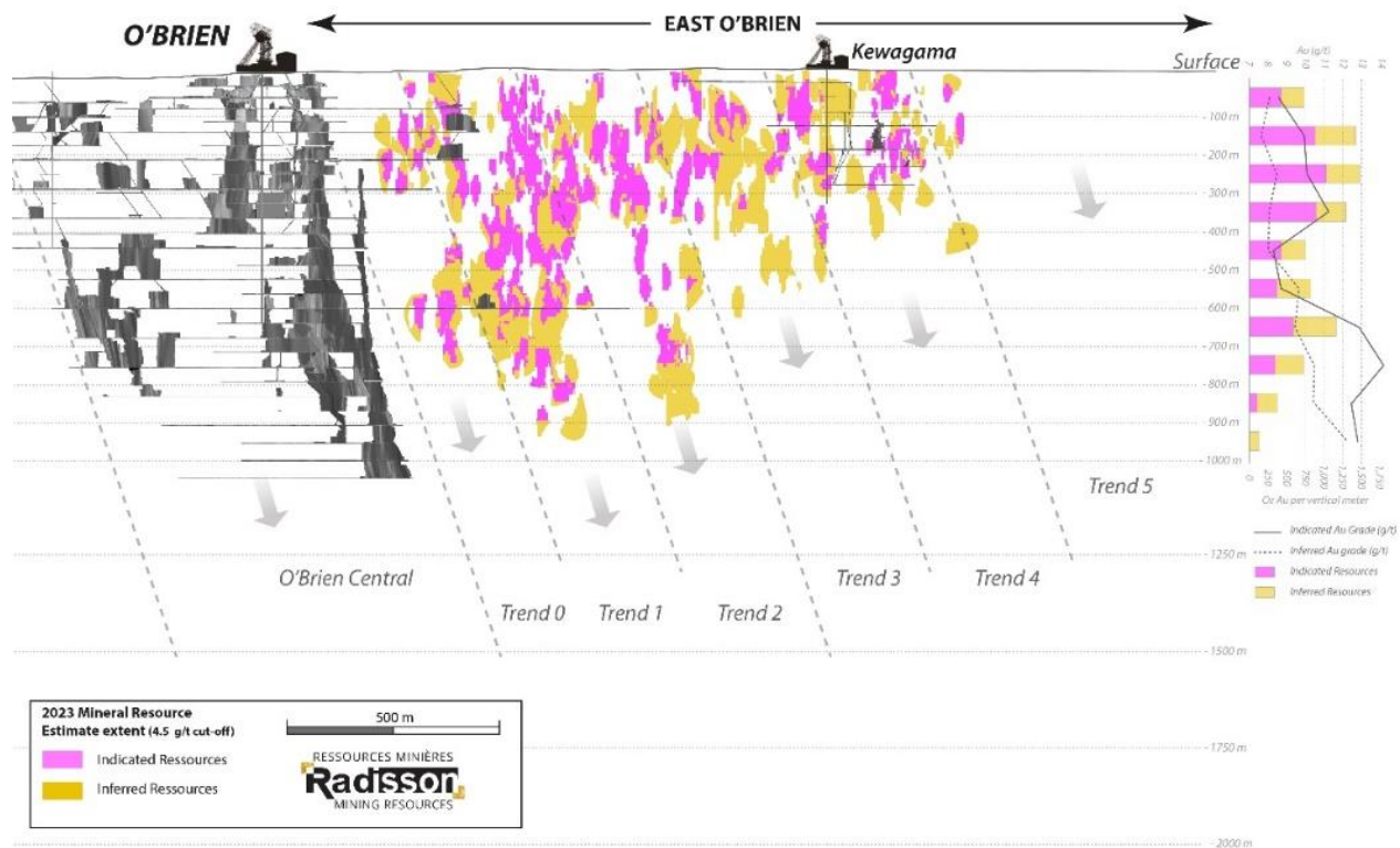
Figure 2. Projet aurifère O'Brien – Vue longitudinale regardant vers le nord - O'Brien Est - Estimation des ressources minérales de 2023 à une teneur de coupe de 4,5 g/t Au
