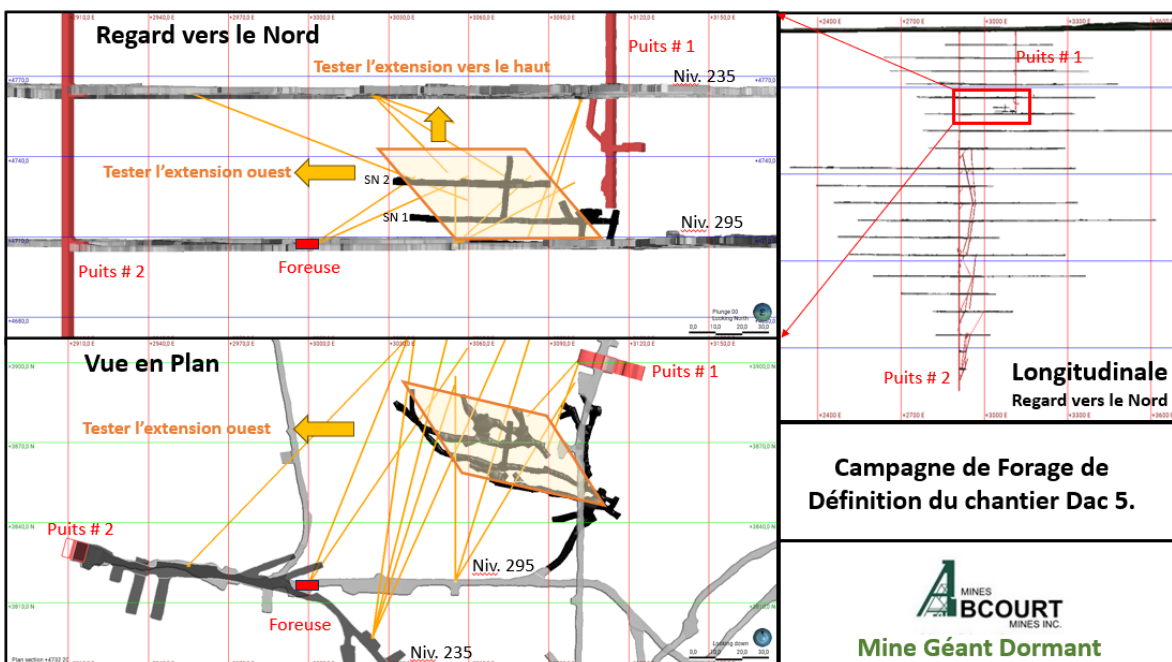
Figure 1 : Campagne de forage de définition, Chantier Dac 5
