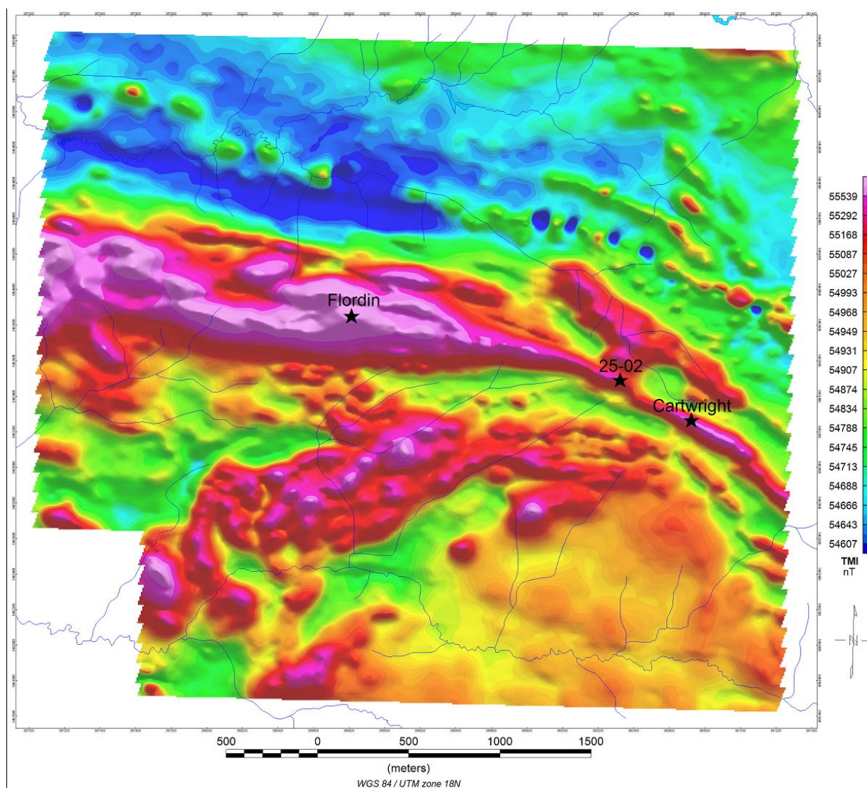
Figure 2 : Carte du champ magnétique total avec la position des décapages Cartwright, 25-02 et le gîte Flordin
