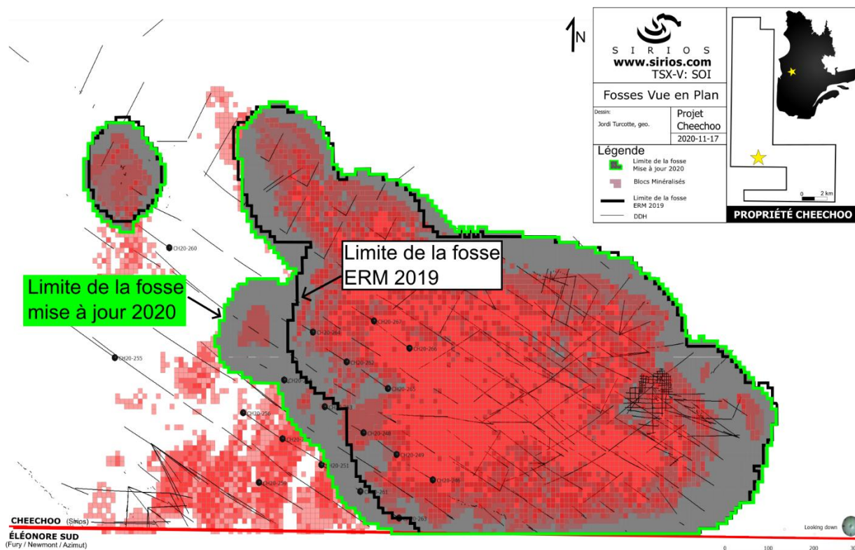
Figure 1 Vue en plan de la fosse conceptuelle. La fosse détournée en noir contient la première estimation des ressources de 1,6 Moz d'or. La fosse en gris et détournée en vert contient la nouvelle estimation des ressources de 1,955 Moz d'or.
