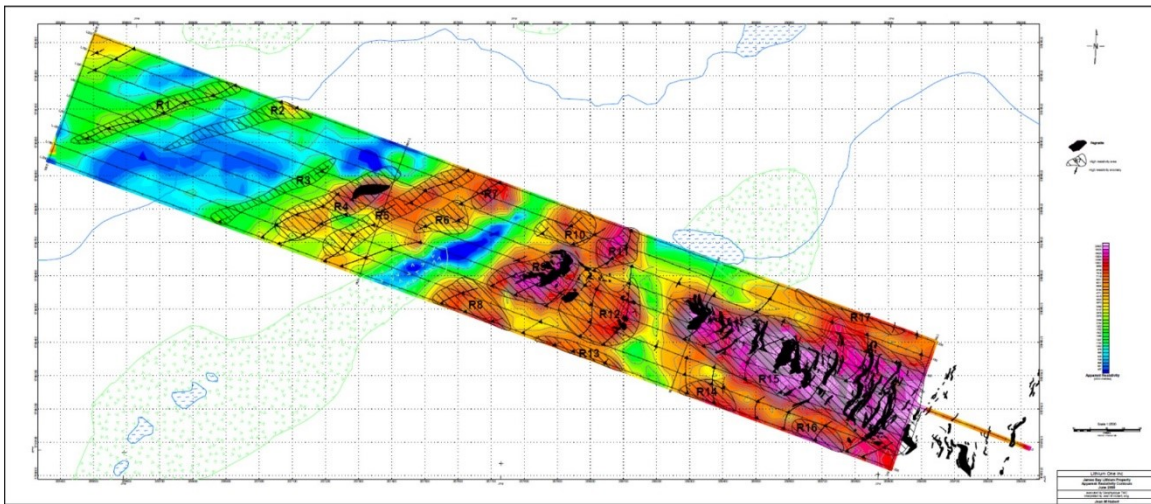
Figure 2. Carte de contour, Résistivité apparente, Galaxy Lithium (2008)
