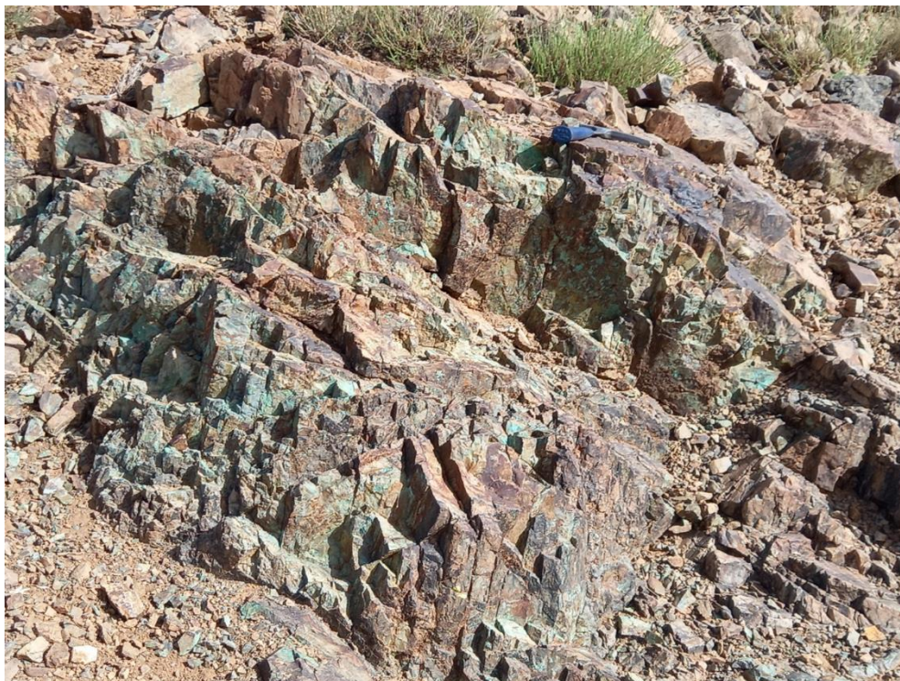
Figure 3 : Affleurement riche en malachite observé dans le cadre de la campagne de cartographie du projet Zgounder Régional
