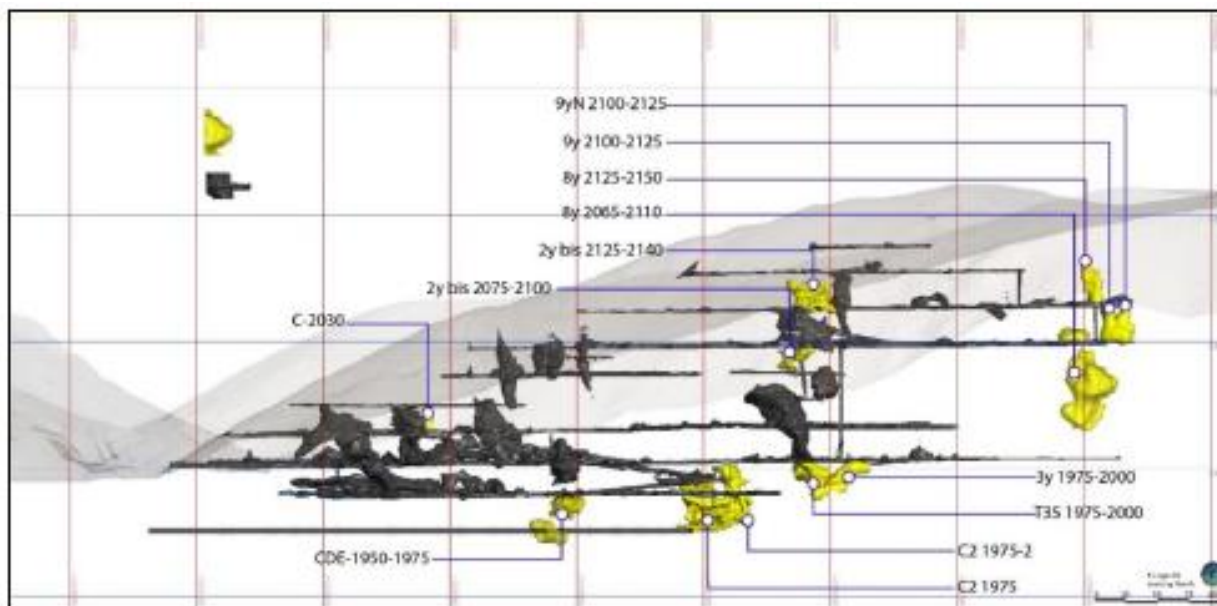
Figure 2 : Section longitudinale à Zgounder, montrant le corps minéralisé 8y 2065-2110 à l'extrémité est du gisement
