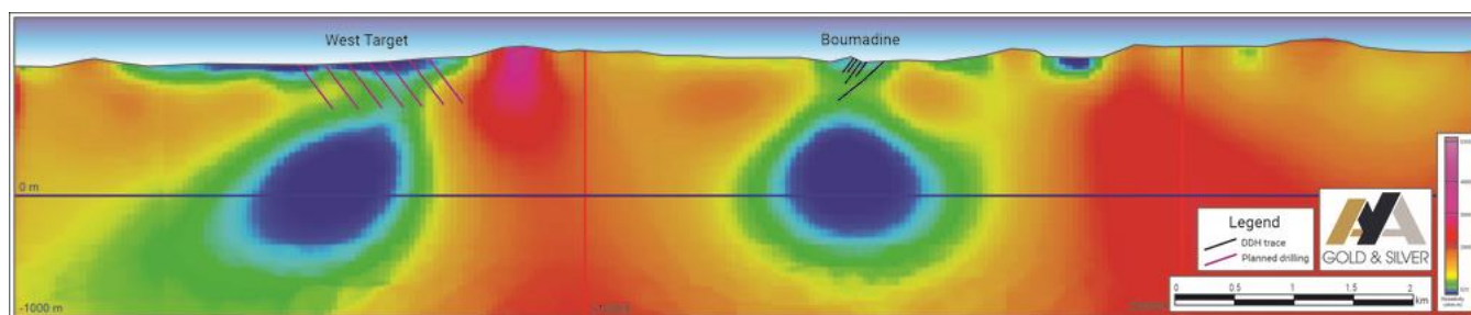
Figure 6 - Section 3476300 montrant l'inversion en 3D et la cible de conductivité à l'ouest
