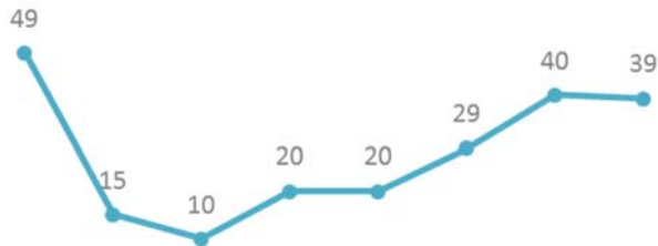
Sélénium
