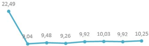
Bismuth
