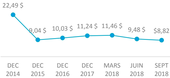
Bismuth
