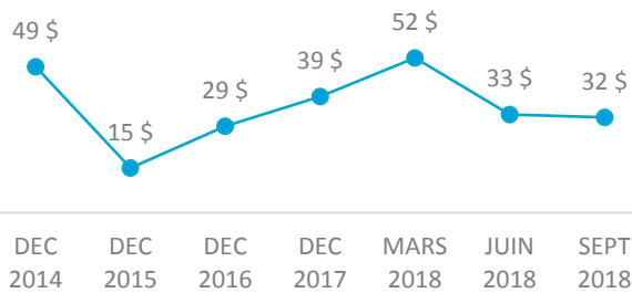
Sélénium
