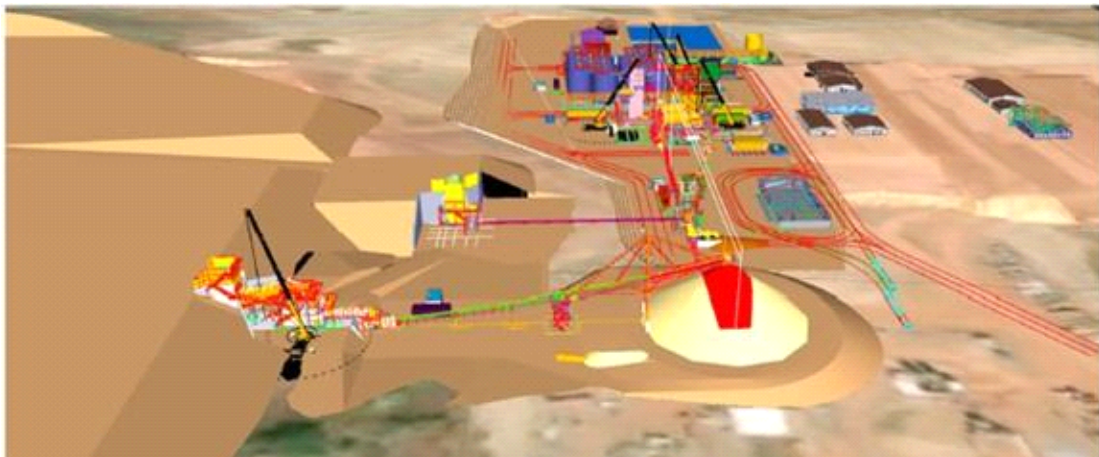
Schéma 2 : Conception actuelle de Primero (achevée à 24 %)
